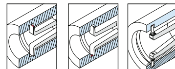
Schneide / Shape R 0,1mm Kugel / Ball Ø 0,6 / 1,0mm Kugel / Ball Ø 1,5 / 2,0mm
